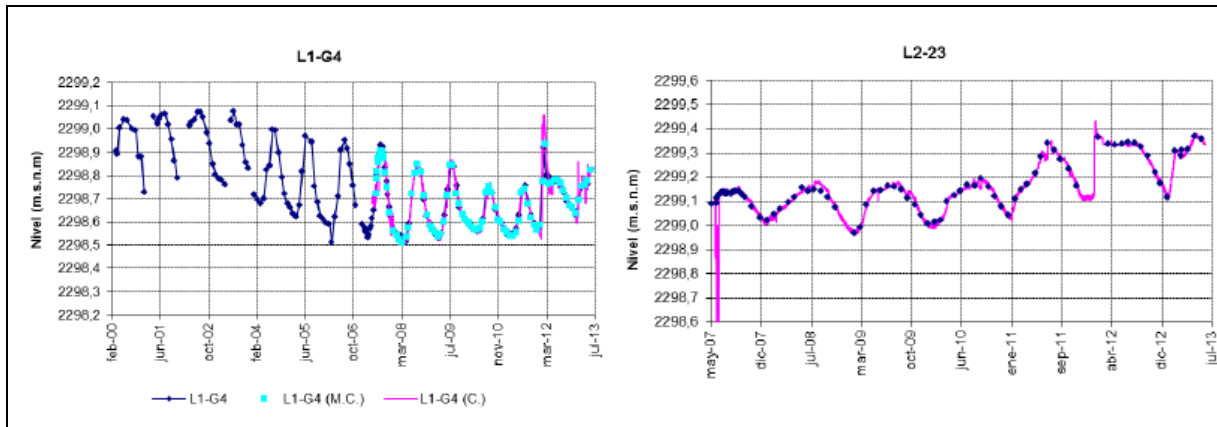
Figura 7-12 Reglilla L1-G4 y pozo L2-23
