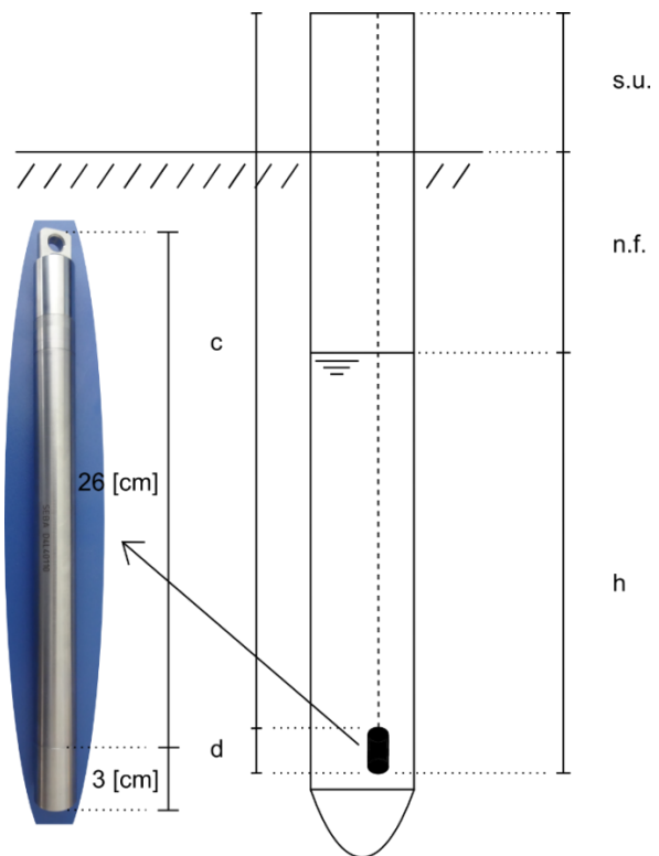
Figura 11-2 Dimensiones características piezómetro
