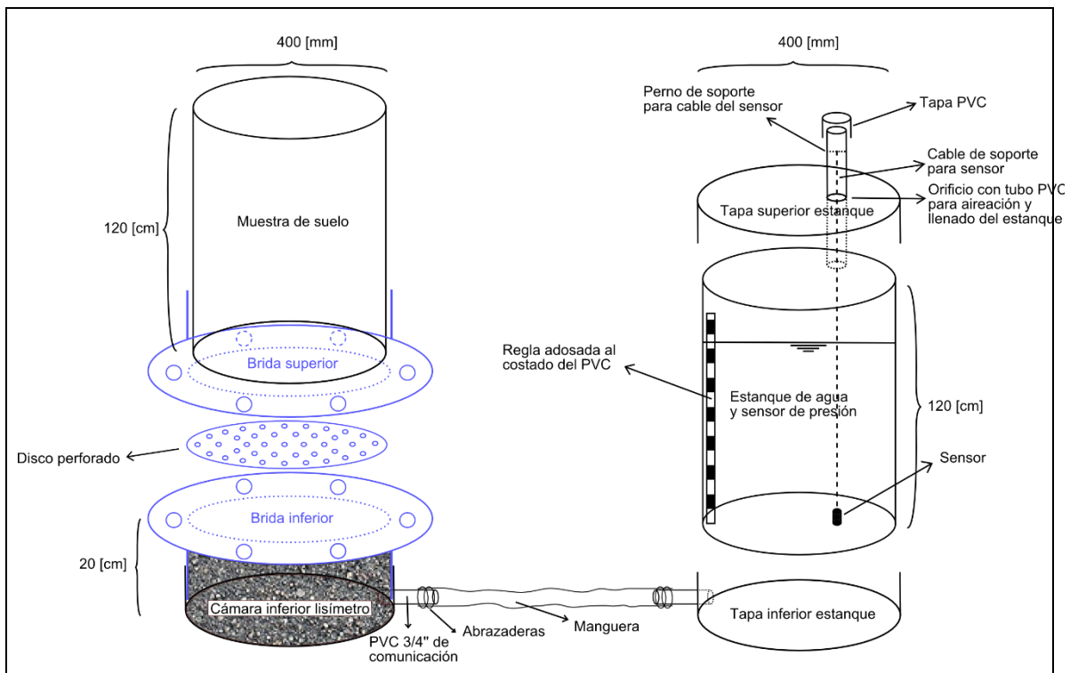
Figura 10-4: Diseño lisímetro
