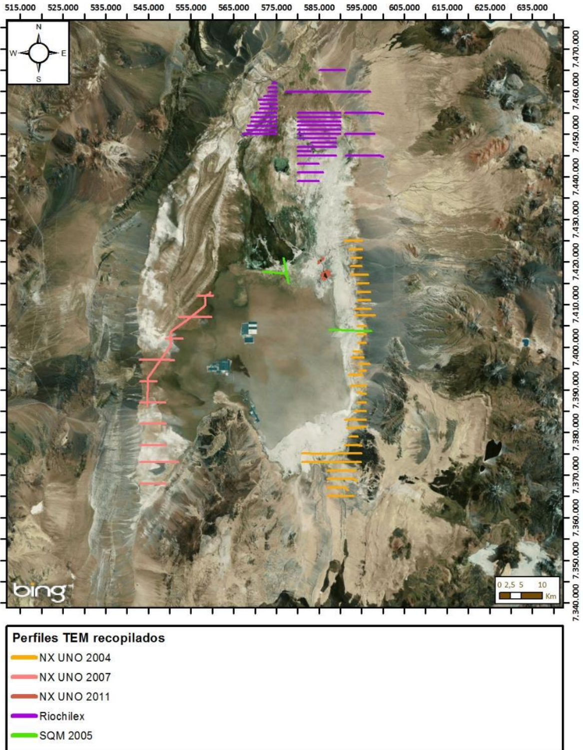
Figura 5-13 Trazado en superficie de los perfiles TEM realizados en el Salar
