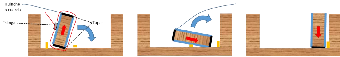
Figura-5: Giro del lisímetro. Flecha roja indica parte superior del suelo.
