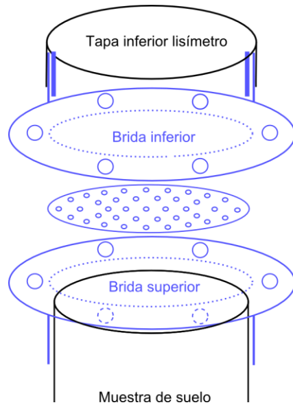
Figura-7: Unión muestra de suelo y tapa inferior.
