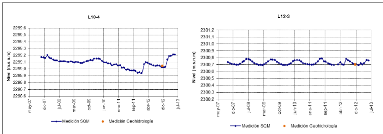
Figura 7-19 Pozo L10-4 y L12-3
