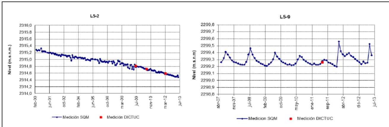
Figura 7-14 Pozos L5-2 y L5-9
