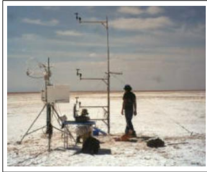
Figura-3 Estación correlación de Eddy (Kampf, 2002)
