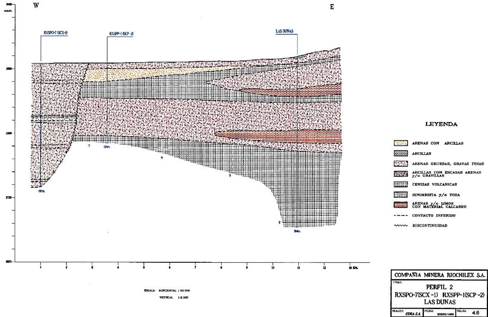
Figura 5-7 Perfil W-E en el norte del Salar elaborado por EDRA (1997)
