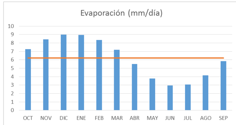
Figura 10-2 Evaporación estación SCL (2002-2012)
