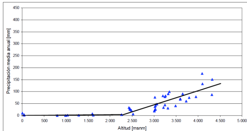
Figura 6-9: Relación Precipitación anual v/s altura. Fuente DGA/DICTUC 2008.
