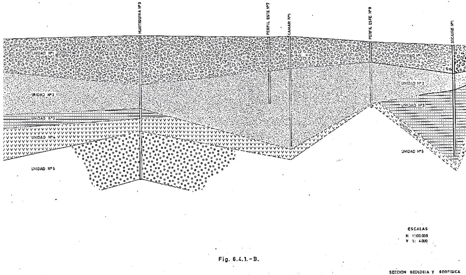
Figura 5-6 Sección Geológica N-S elaborada por Díaz del Río, et al. (1972). Continuación.
