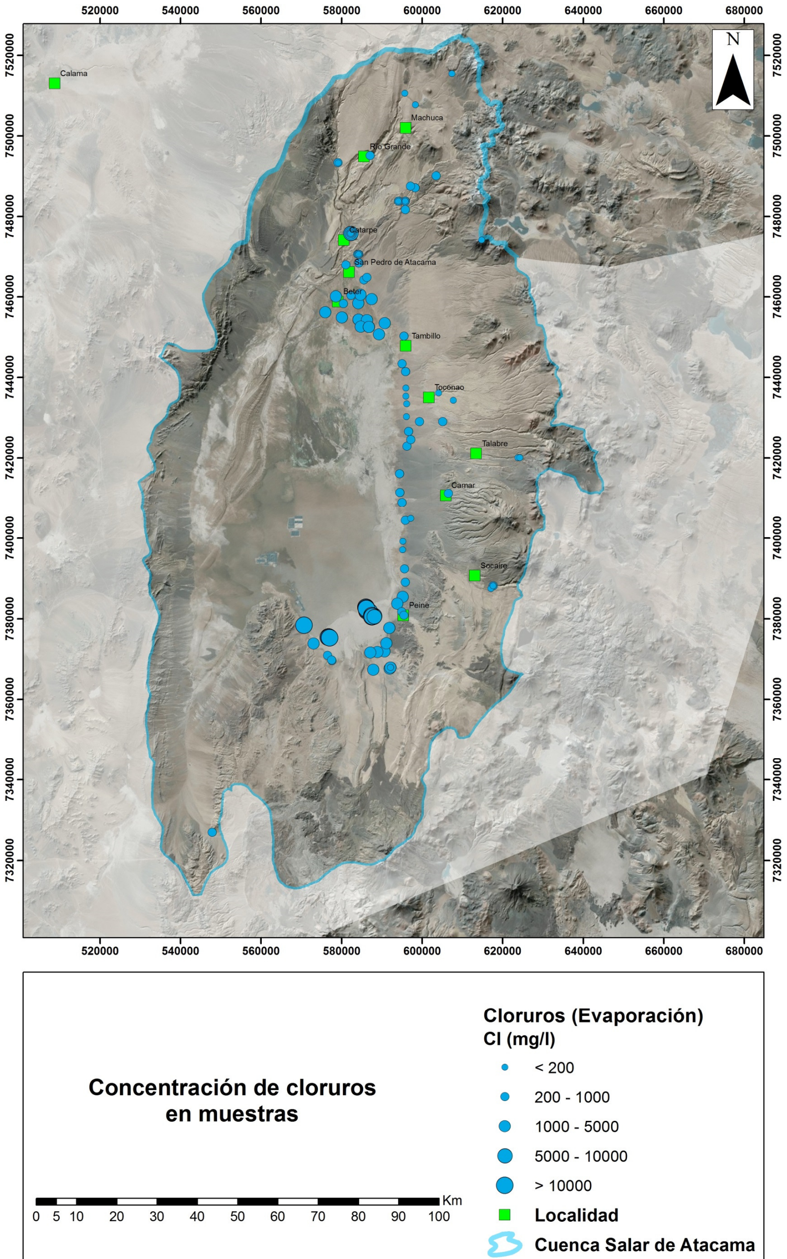
Figura 8-2 Concentración de cloruro (en mg/l) de las muestras
