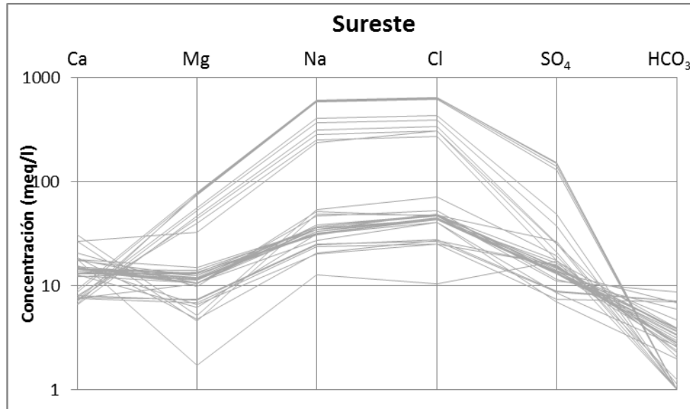
Figura 8-9 Diagrama de Schöeller con las muestras del sector sureste del Salar de Atacama.
