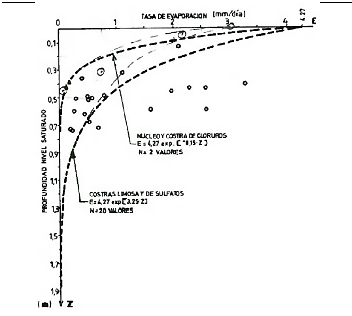
Figura 9-3 Curva evaporación v/s profundidad DGA, 1986.
