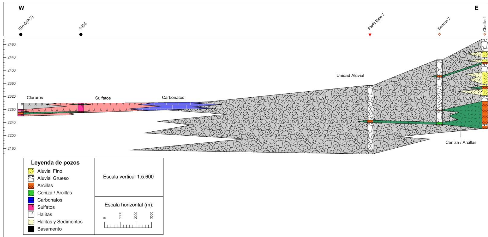
Figura 5-10 Perfil geológico WE2
