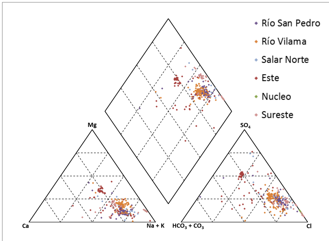
Figura 8-10 Diagrama de Piper con todas las muestras analizadas.
