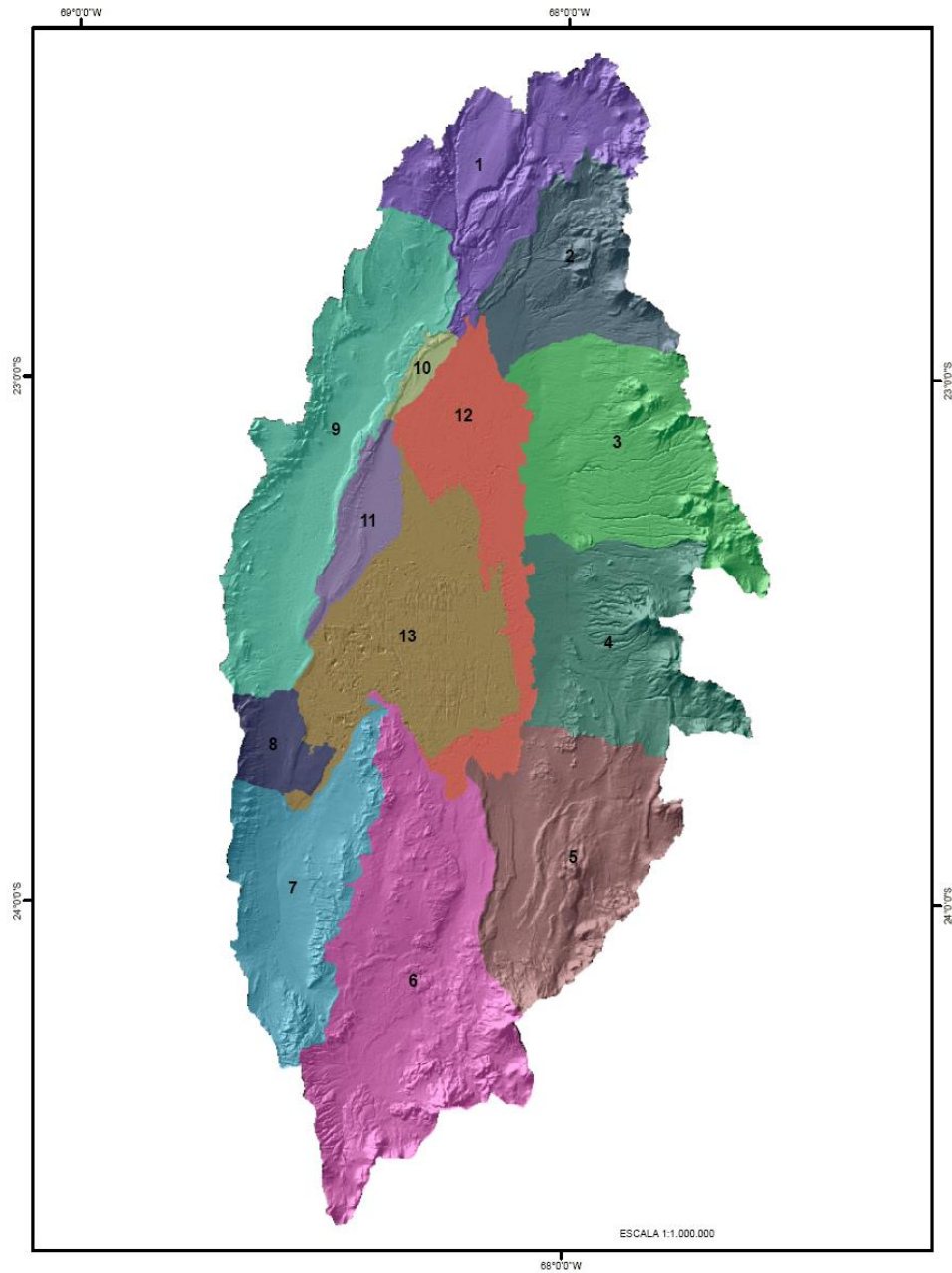
Figura 6-5: Subcuencas cuenca del Salar de Atacama. Fuente: DGA/GCF 2010.
