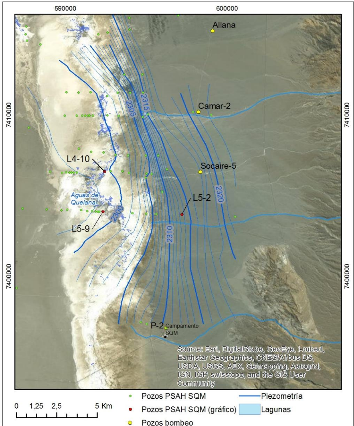
Figura 7-13 Piezometría Aguas de Quelana (modificado de Fock, 2009)
