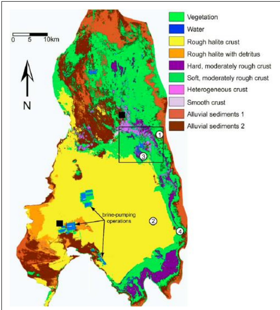
Figura 9-4 Zonación superficie Kampf, 2006
