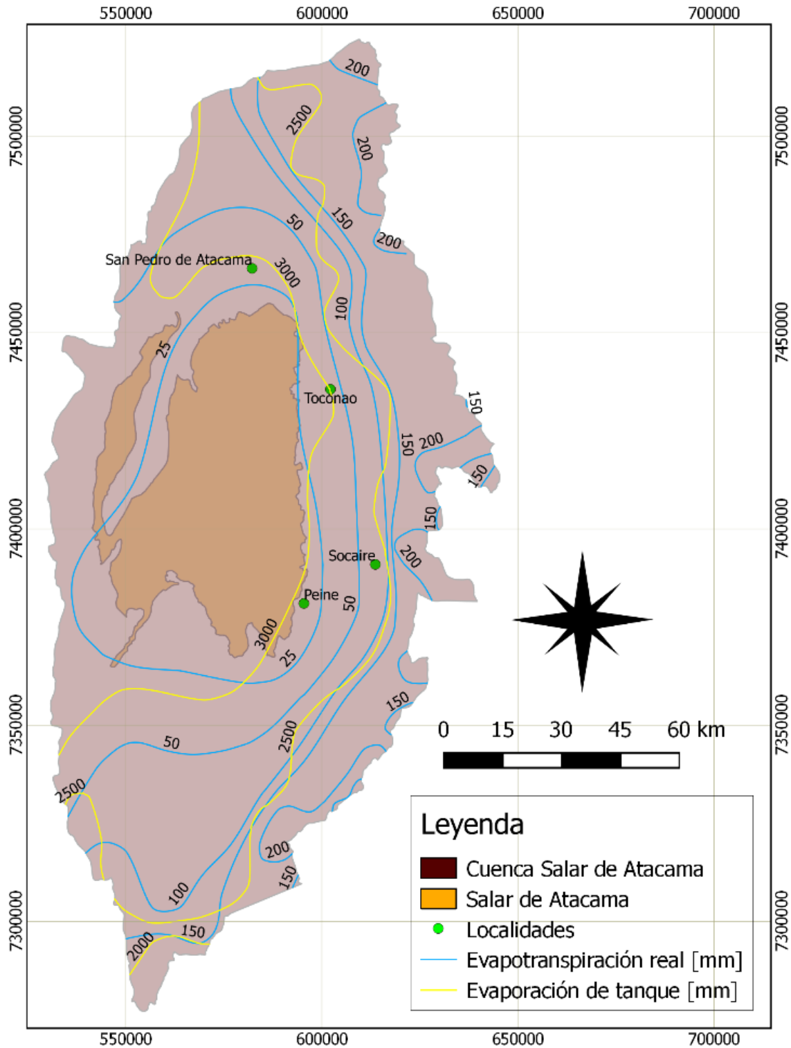
Figura 6-12: Isolíneas de evaporación. Fuente: Balance Hídrico Nacional, 1987.
