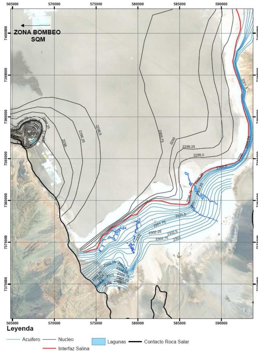
Figura 7-17 Piezometría 2012 sector sur (Anexo 3 de EIA de RWL)
