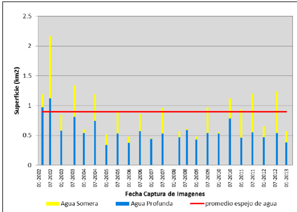
Figura 7-21 Superficie lagunas sector sur (PAT MEL 2013).
