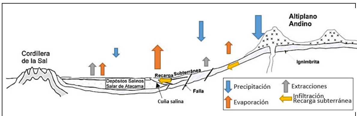
Figura 9-9: Modelo conceptual (modificado de DICTUC, 2004)
