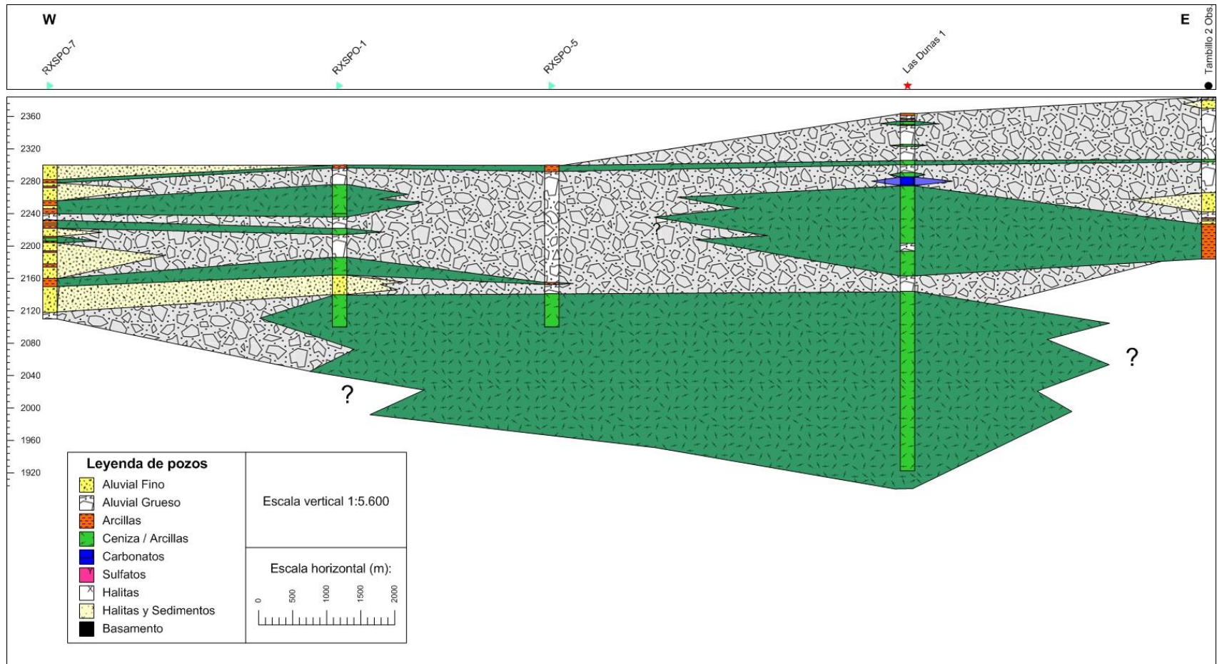
Figura 5-11 Perfil geológico WE3
