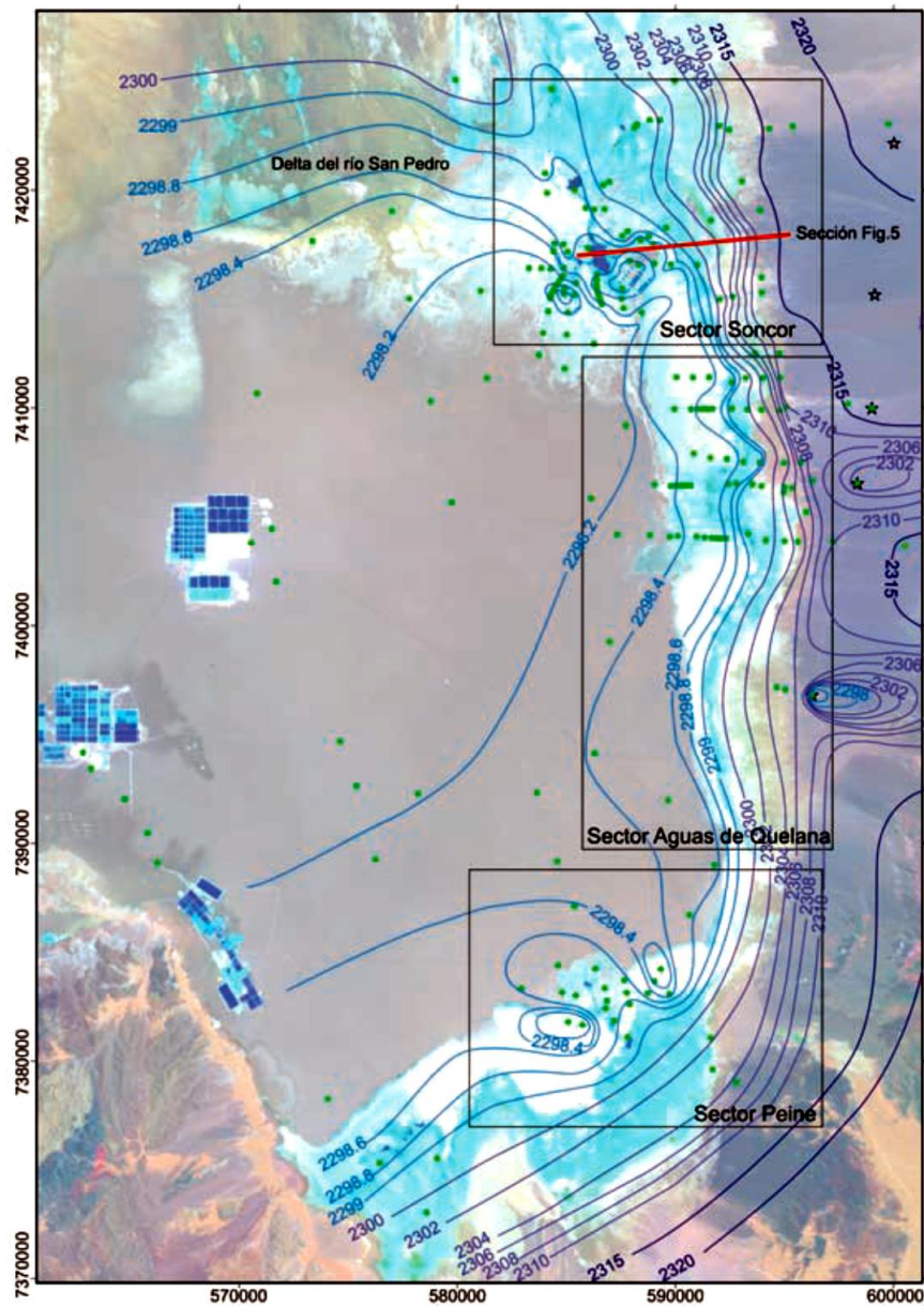
Figura 7-7 Piezometría borde oriental (Salas et al., 2010)
