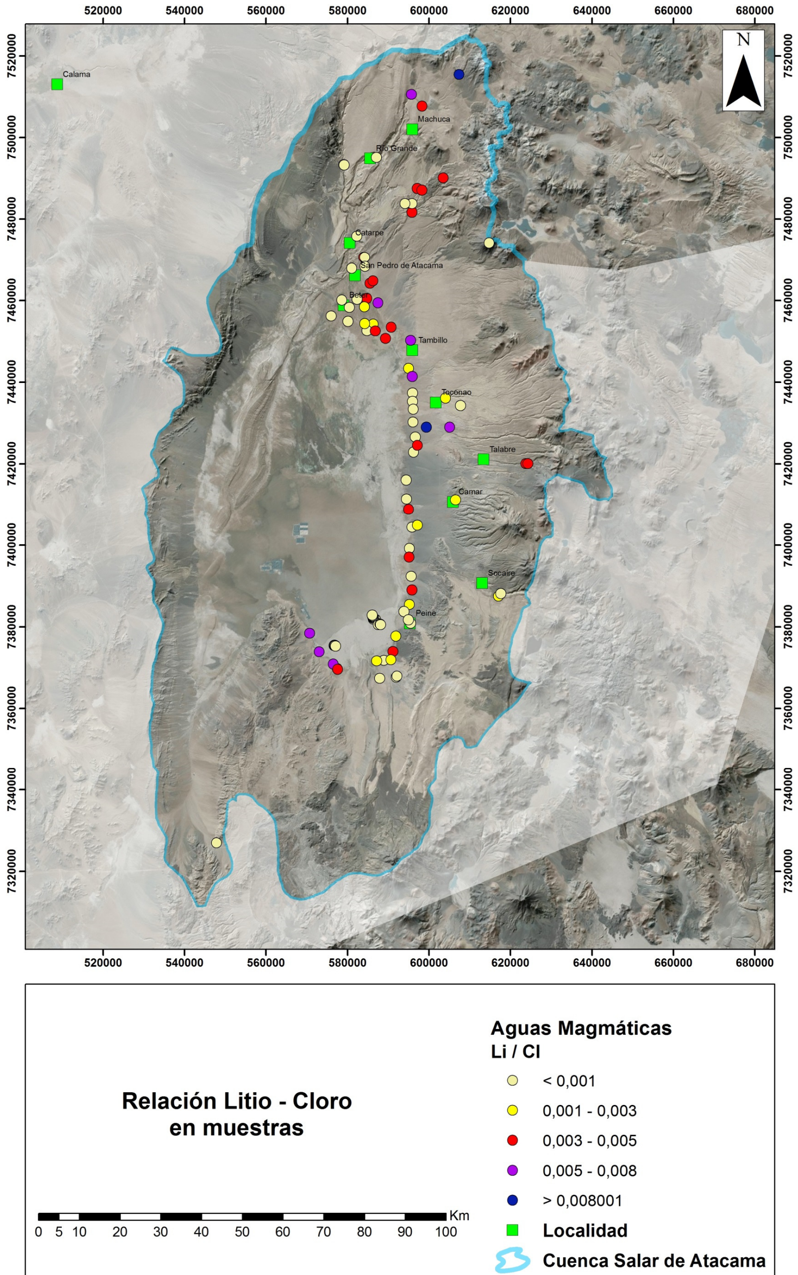
Figura 8-3 Relación Li/Cl de las muestras
