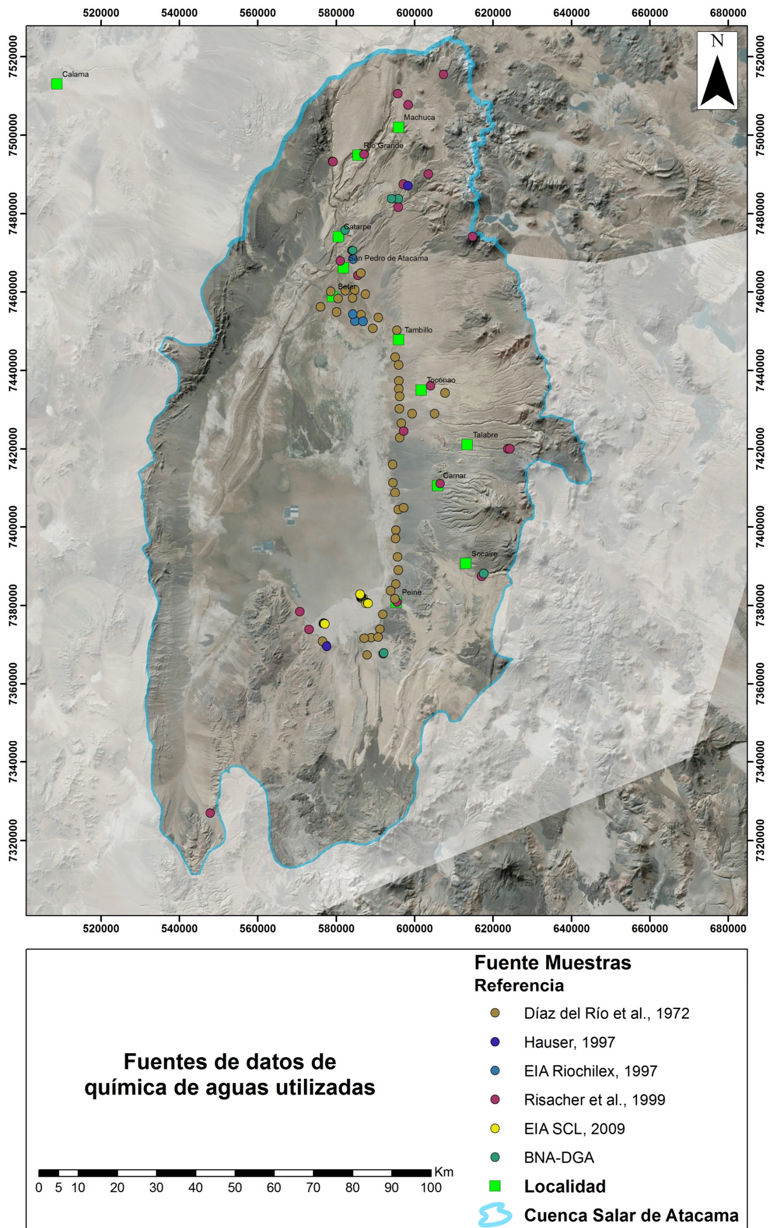
Figura 8-1: Ubicación y fuente de las muestras utilizadas en este trabajo.
