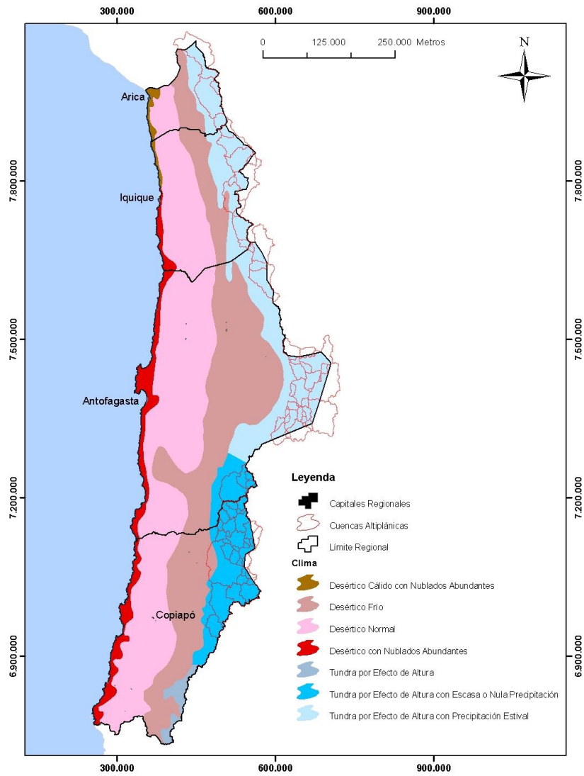
Figura 6-2: Clima de las regiones XV, I, II y III de Chile. Fuente DGA/DICTUC 2008.
