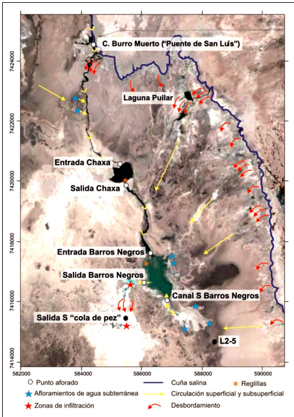
Figura 7-11 Sistema Soncor (Salas et al., 2010)
