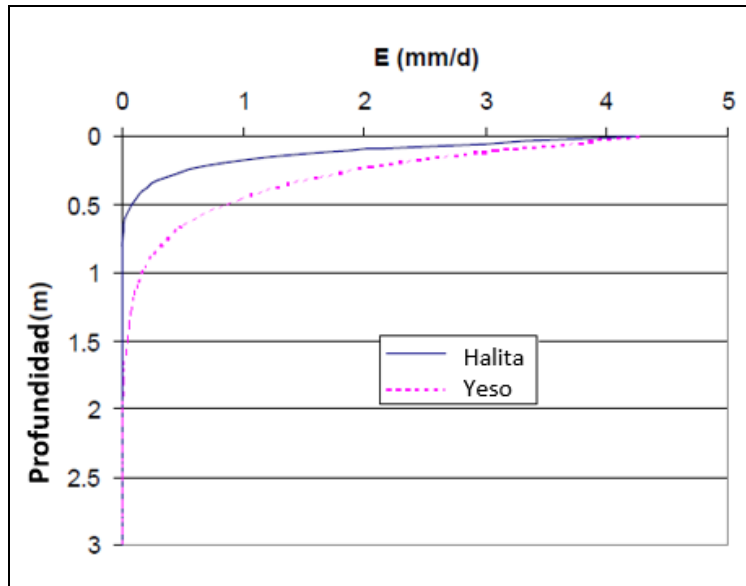
Figura 10-1 Evaporación v/s profundidad. Modificado de Kampf, 2002
