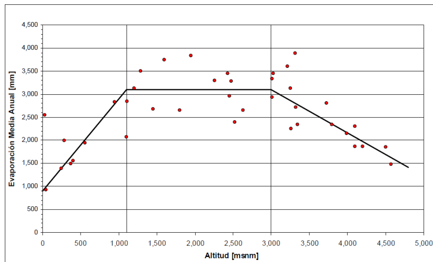
Figura 6-13: Gradiente evaporación media anual regiones de la XV a la III.
