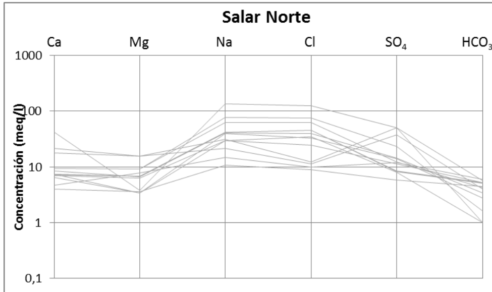
Figura 8-6 Diagrama de Schöeller con las muestras de la parte norte del Salar de Atacama
