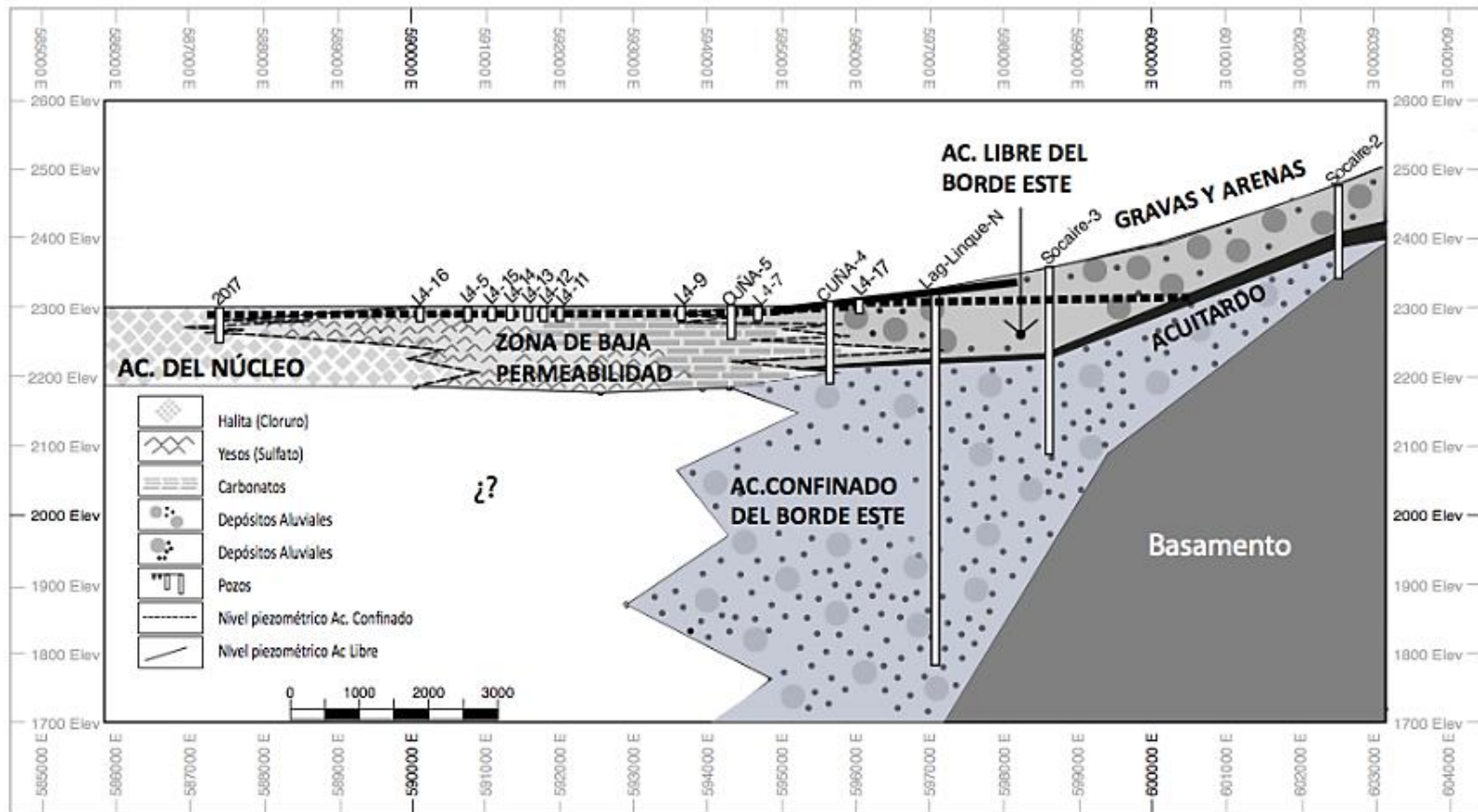
Figura 7-6 Perfil hidrogeológico del borde oriental del Salar de Atacama
