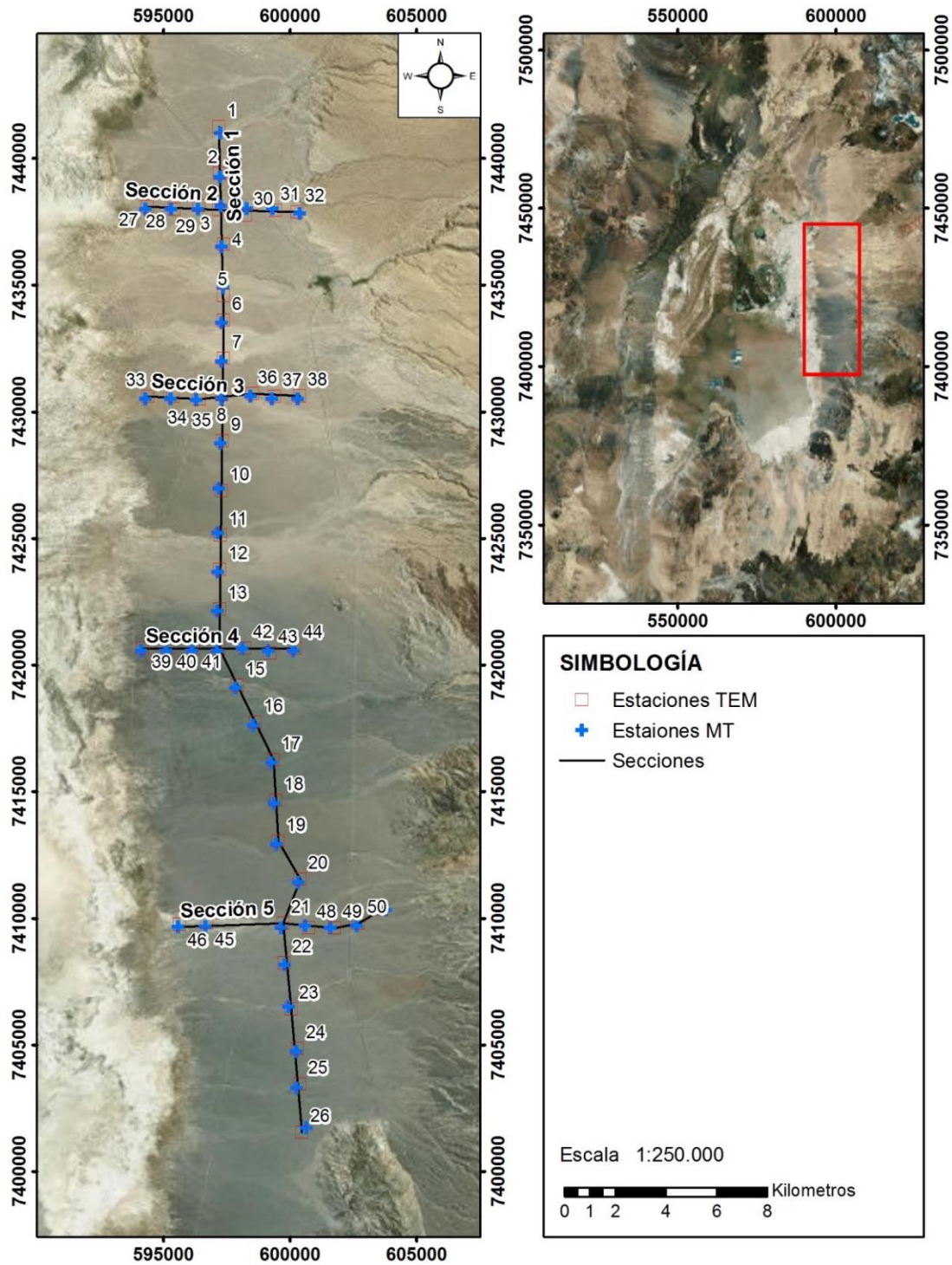
Figura 5-14 Trazado en superficie de los perfiles TEM y MT realizados en el borde este Salar
