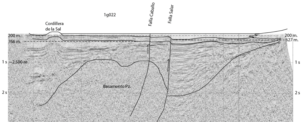
Figura 5-12 Perfil de refracción sísmico 1g022. Fuente: Arriagada et al. (2006)
