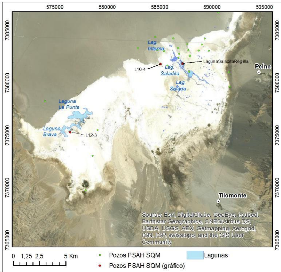
Figura 7-18 Pozos L10-4 y L12-3 y Regilla Saladita
