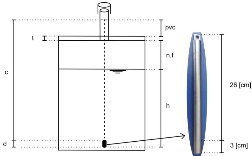
Figura 11-1: Medidas estanque.
