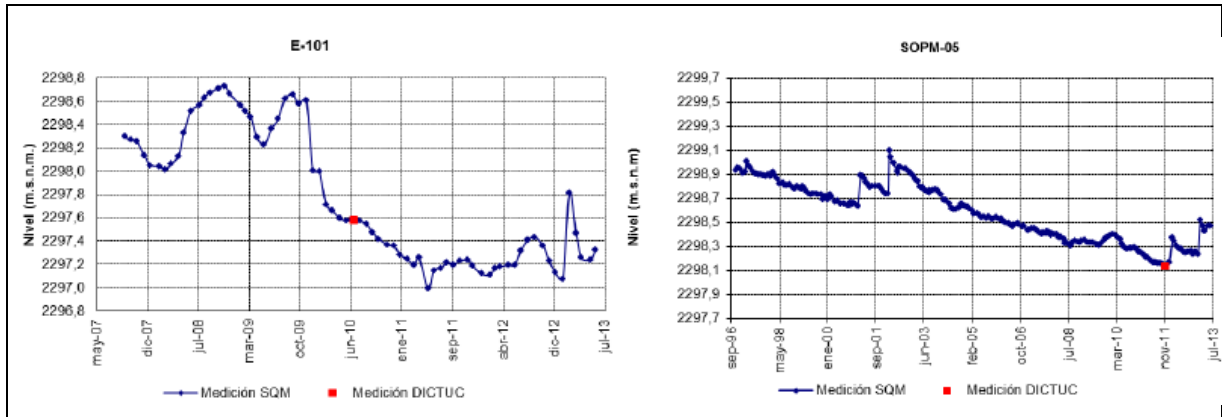
Figura 7-23 Pozos E-101 y SOPM-05
