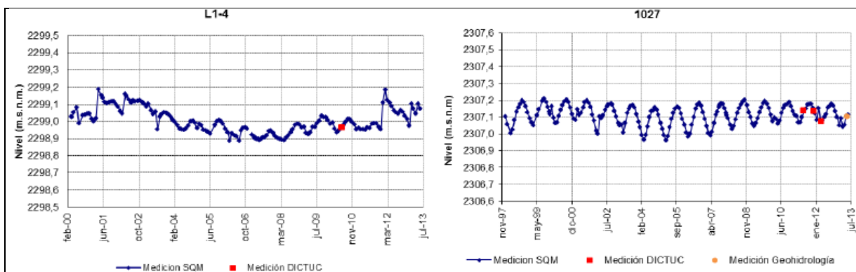
Figura 7-10 Pozos L1-4 y 1027 (PSAH SQM 2013)
