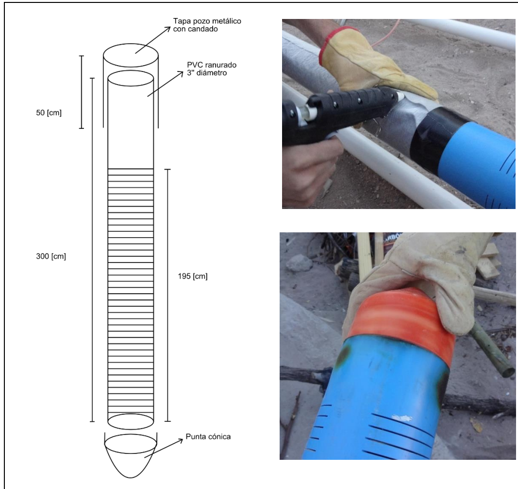
Figura 10-8 Construcción piezómetro
