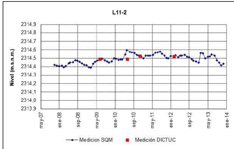
Figura 7-4 Nivel piezómetro L11-2 (PSAH SQM 2014)
