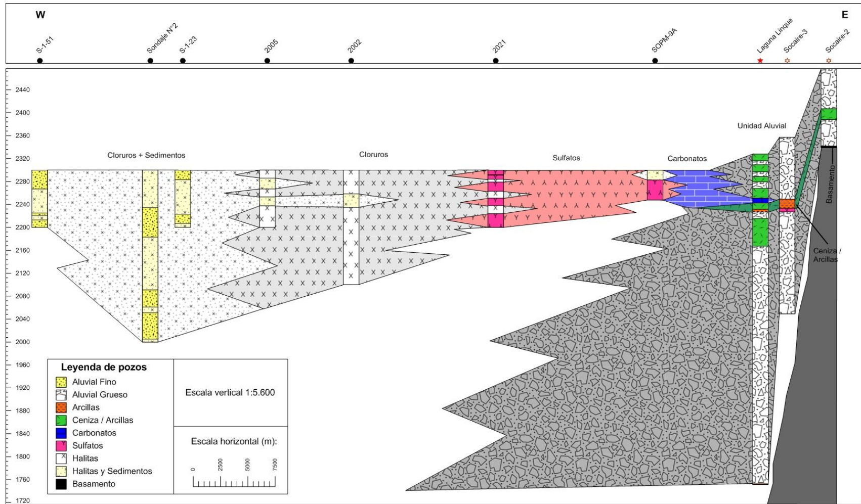
Figura 5-9 Perfil geológico WE1
