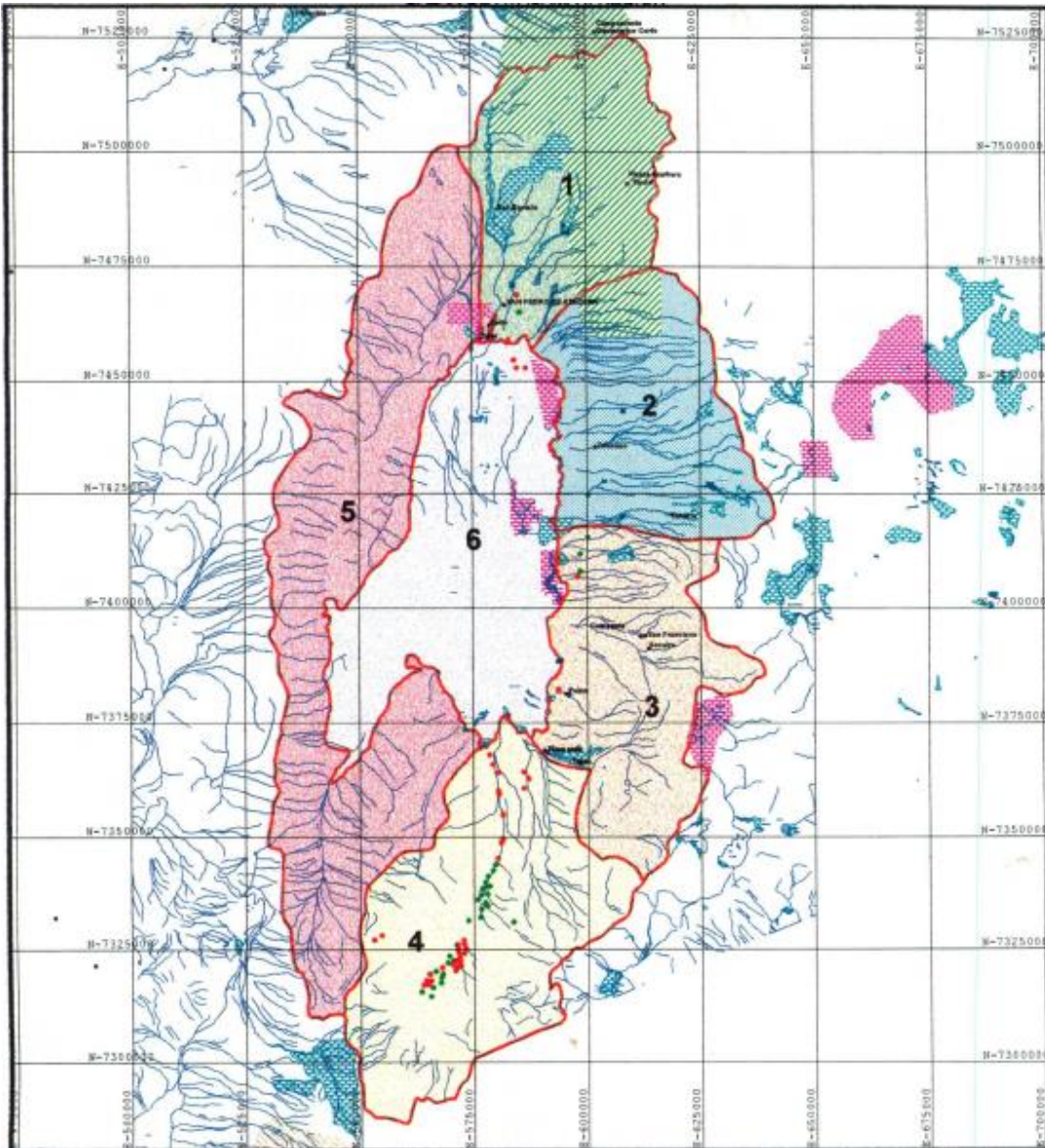
Figura 9-1: Delimitación de subcuencas Minuta 60, 1998.
