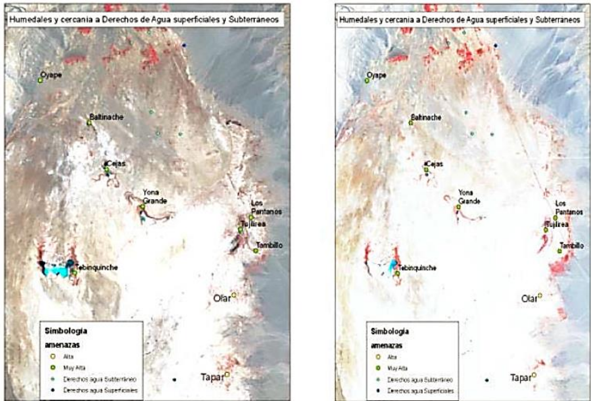
Figura 7-5 Lagunas sector norte (CIREN, 2011)
