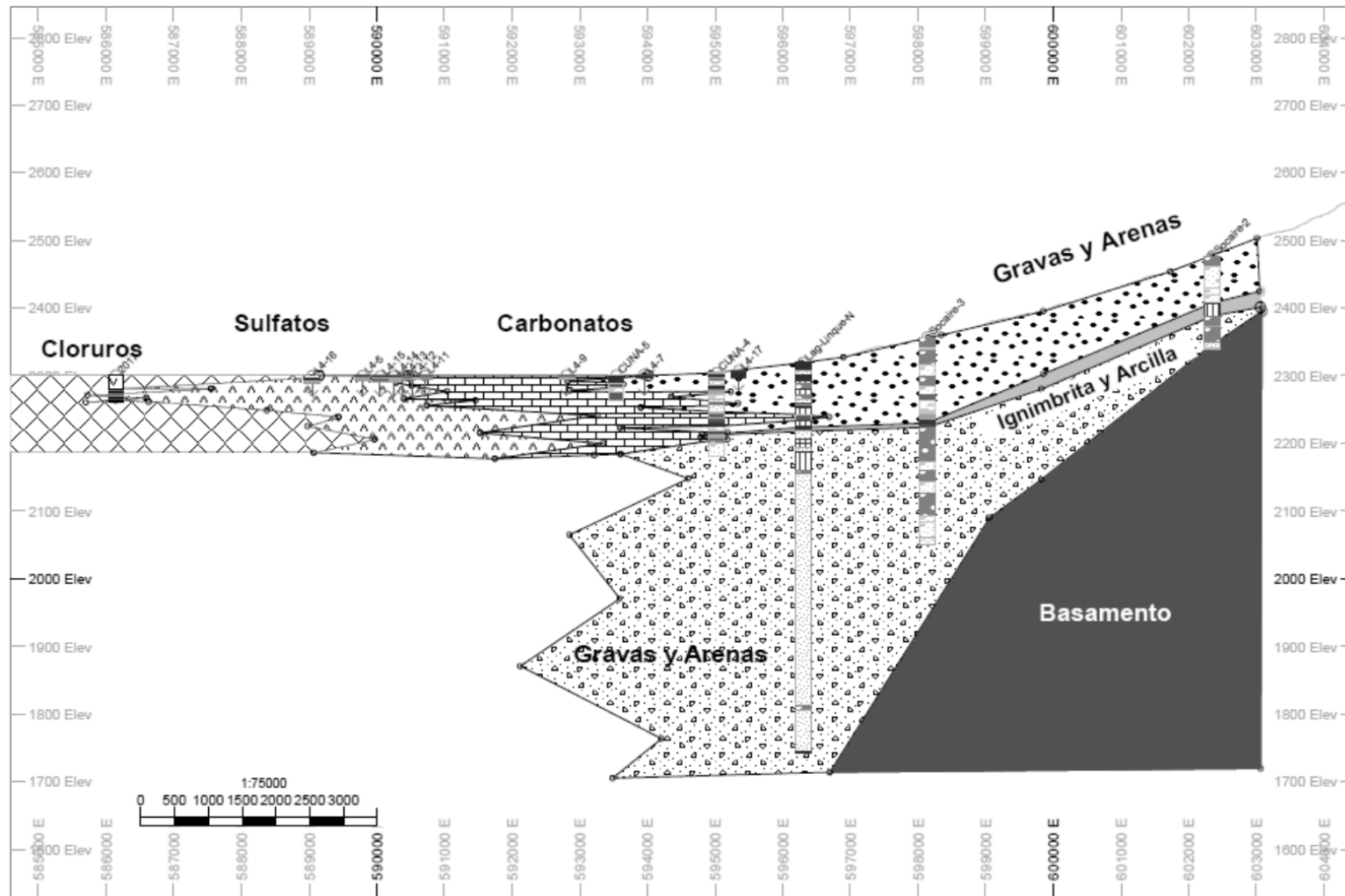
Figura 5-4 Perfil W-E en elaborado por Fock 2011. Fuente: Fock (2011).
