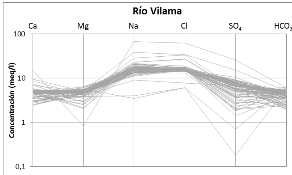
Figura 8-5 Diagrama de Schöeller con las muestras del río Vilama
