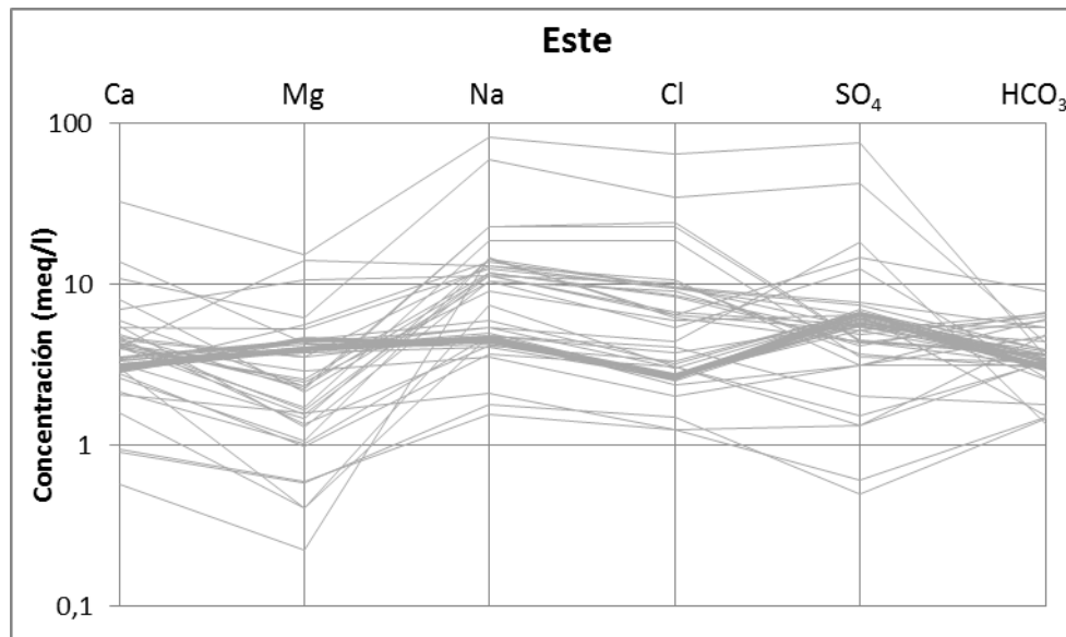
Figura 8-8 Diagrama de Schöeller con las muestras del borde este del Salar de Atacama
