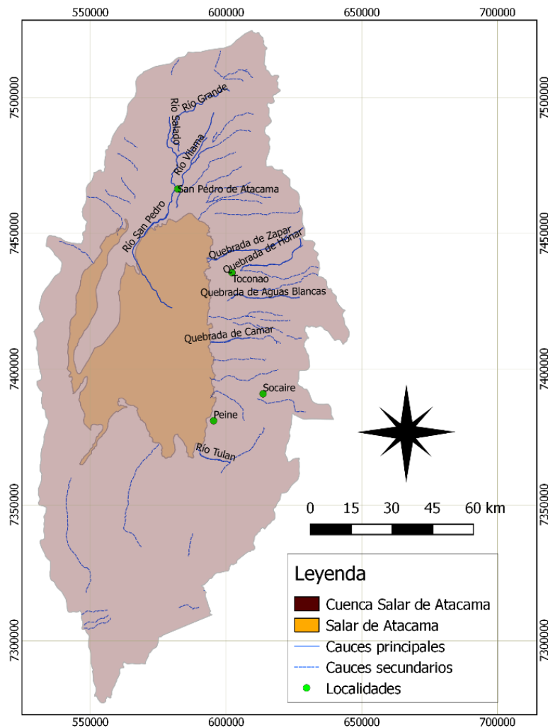
Figura 6-4: Hidrografía cuenca del Salar de Atacama.
