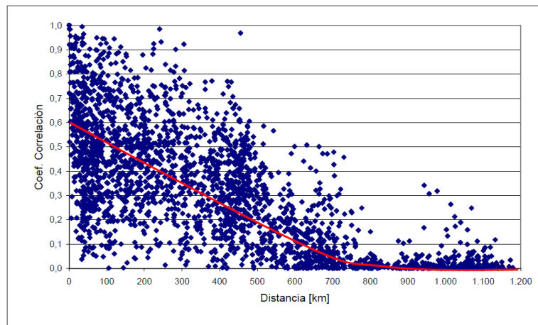
Figura 6-10: Relación coeficiente de correlación de la precipitación media anual entre 2 estaciones v/s la distancia entre ellas. Fuente DGA/DICTUC 2008.
