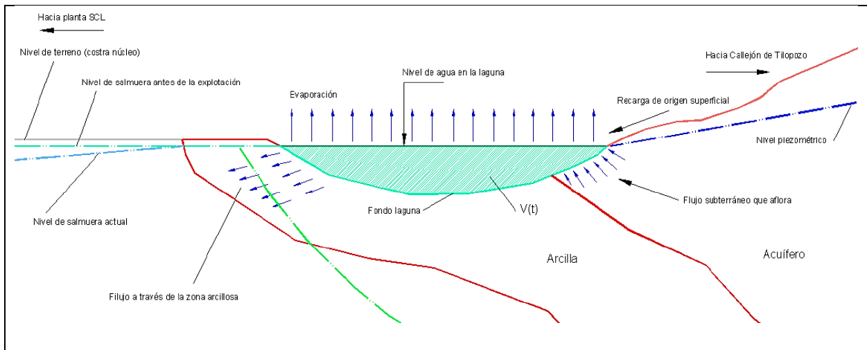
Figura 7-16 Diagrama hidrogeología sector sur (modificado de EIA RWL)
