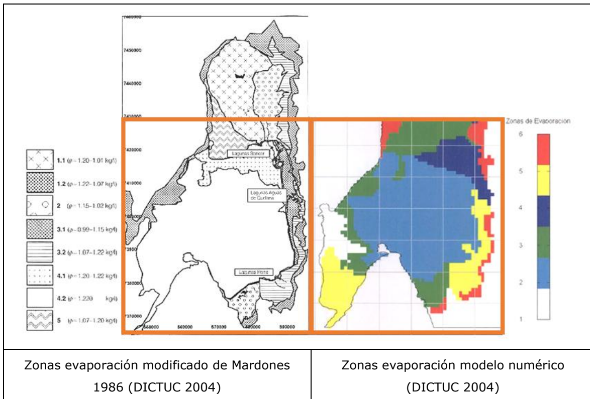
Figura 9-6 Zonas evaporación DICTUC 2004 (no están a la misma escala)
