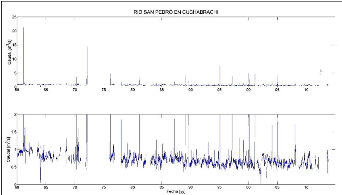
Figura 6-11: Serie de caudales medios diarios Río San Pedro en Cuchabrachi.
