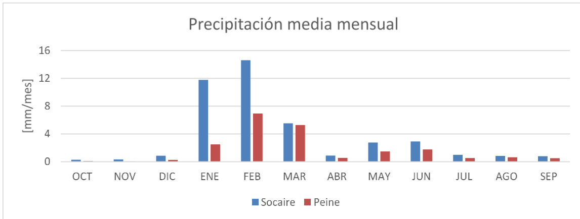
Figura 6-1: Precipitaciones medias mensuales cuenca del Salar de Atacama.
