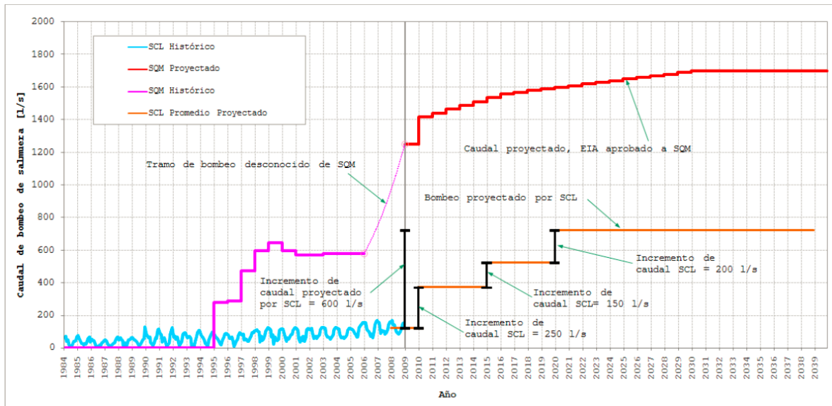
Figura 9-8 Extracciones de salmuera en el núcleo del Salar.
