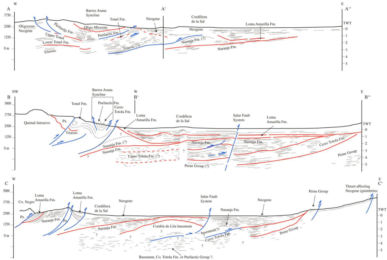
Figura 5-2 Secciones geológicas oeste-este presentadas por Arriagada, et al., (2006). Se presenta ubicación de las secciones en Figura 5-1. Fuente: Arriagada, et al. (2006)
