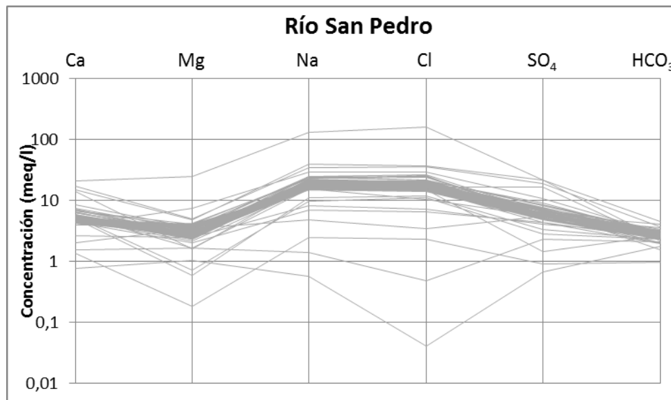
Figura 8-4 Diagrama de Schöeller con las muestras del río San Pedro
