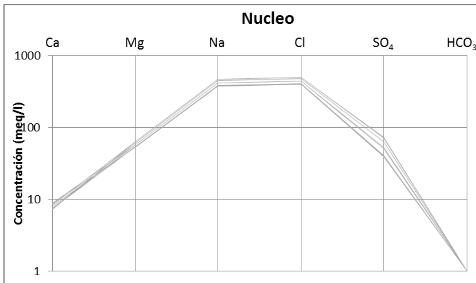
Figura 8-7 Diagrama de Schöeller con las muestras del núcleo del Salar de Atacama
