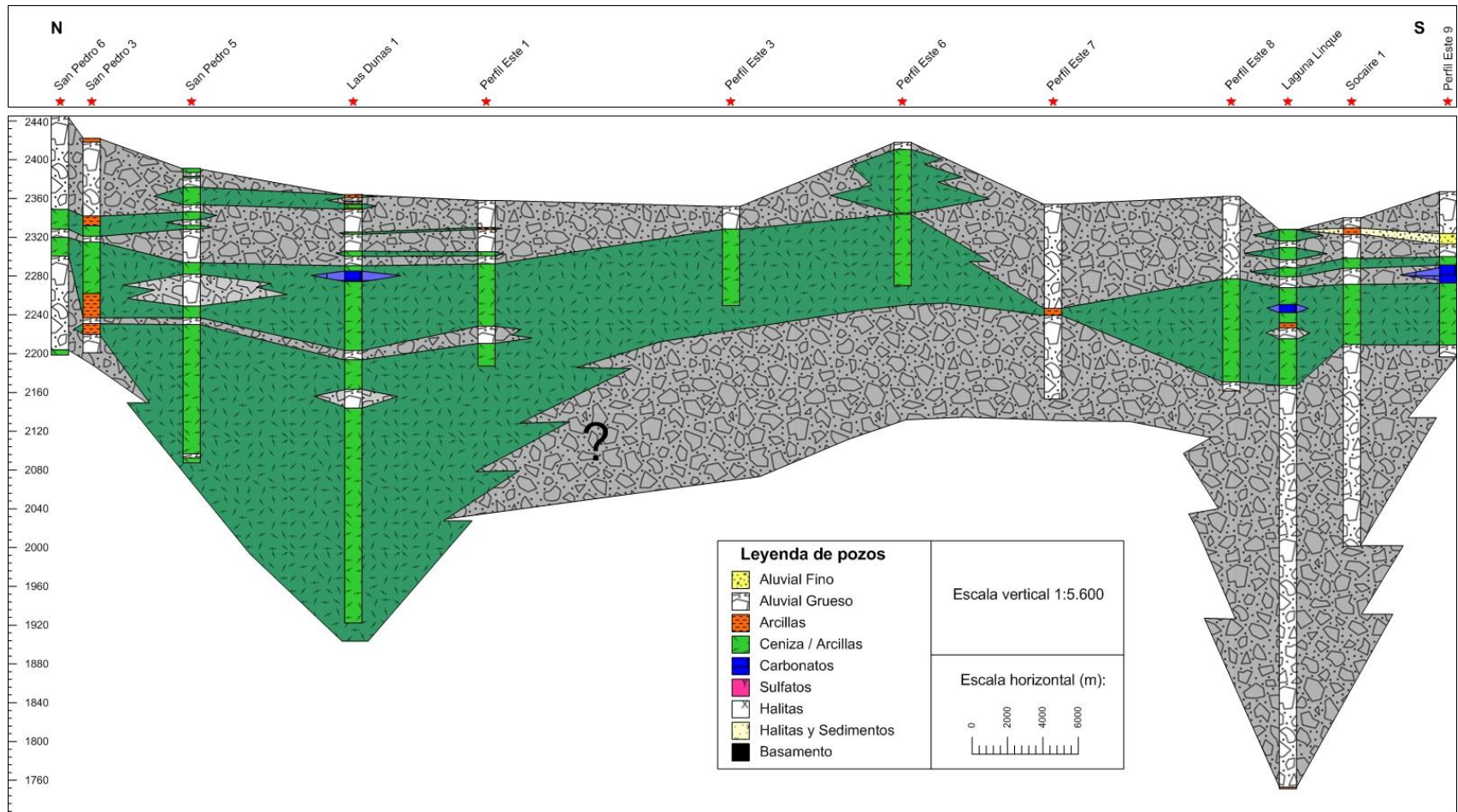
Figura 5-8 Perfil geológico N-S
