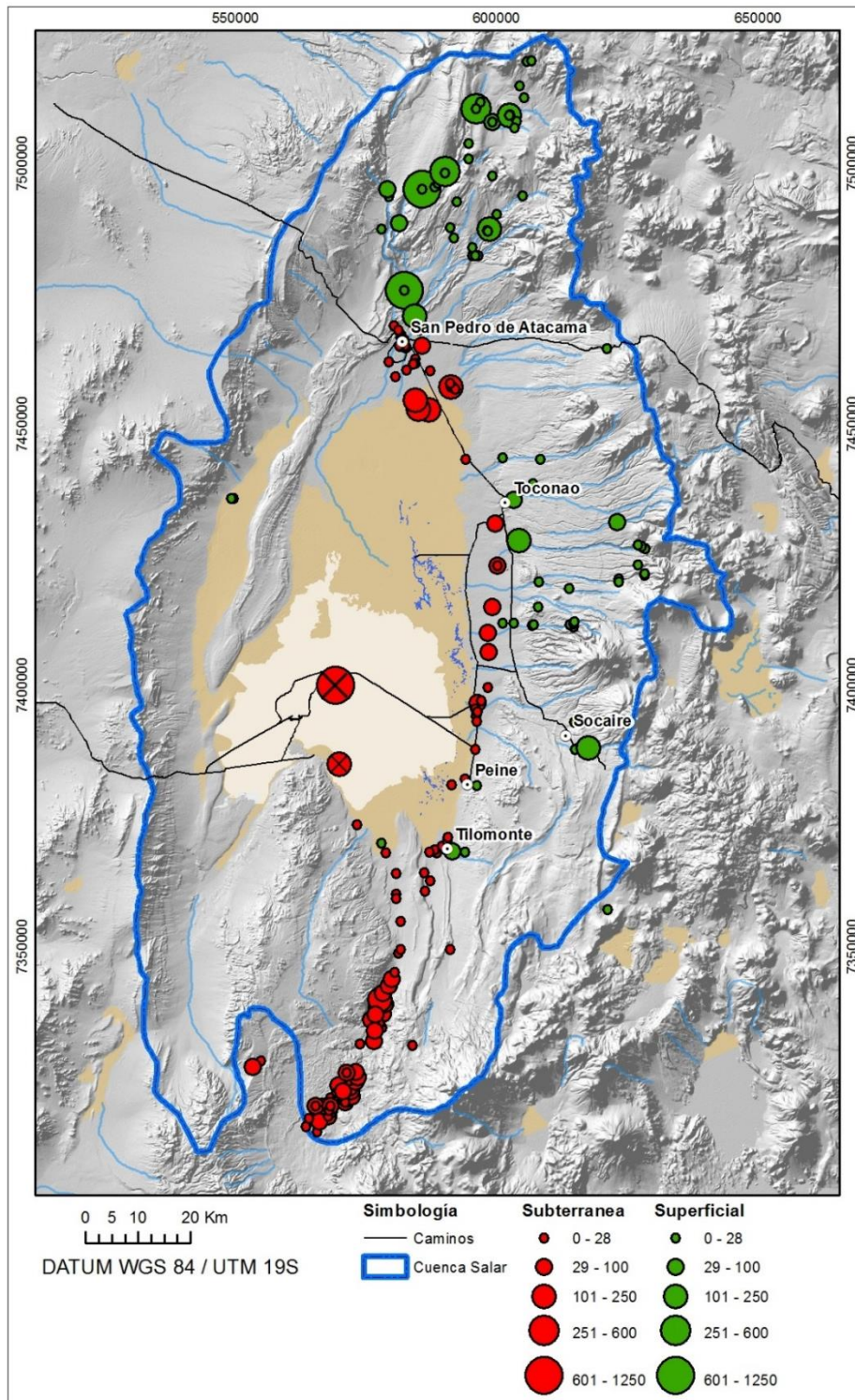
Figura 9-7 Derechos otorgados. Modificado de DGA/CGF, 2010. Las extracciones en el núcleo de RWL y SQM se señalan con una X y corresponden extracciones mineras.
