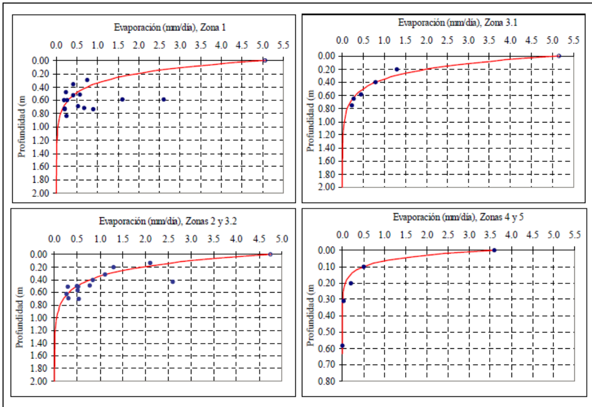
Figura 9-5 Curvas evaporación Muñoz et al., 2004
