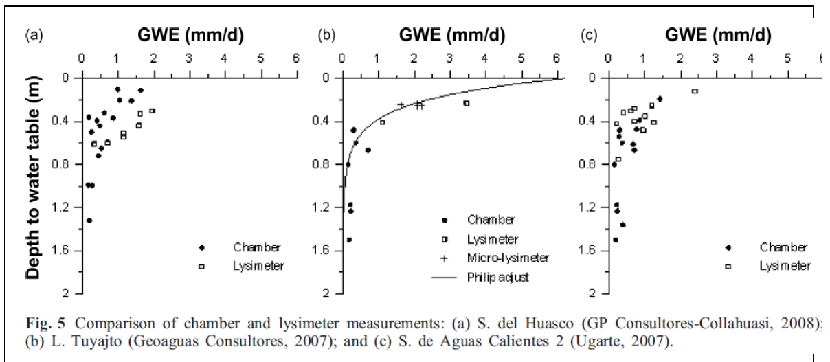
Figura-5 Comparación instrumentos Johnson et al., 2010
