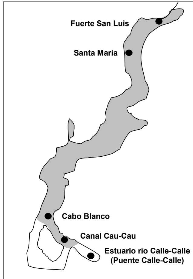
Figura 82. Ubicación aproximada de las estaciones de muestreo en el río Cruces (sectores Fuerte San Luis, Santa María y Cabo Blanco), canal marealed Cau-Cau y estuario del río Calle-Calle. El color gris señala la extensión aproximada de las aguas color marrón durante la mayor parte de este estudio.
